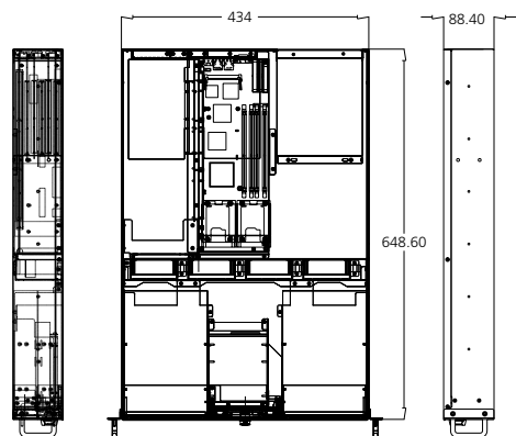
顶部视图
